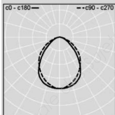
Actison RWS 280 courbe des intensités lumineuses
