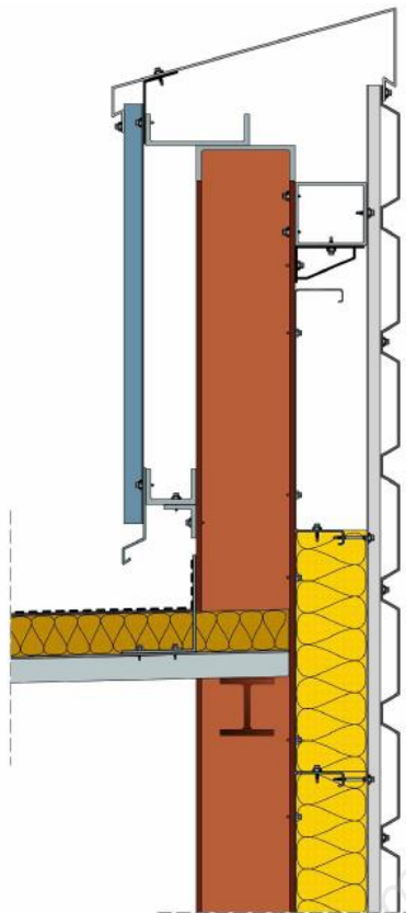
Figure 26 - Détail du haut de Bardage Horizontal Exemple de solution avec ossature intermédiaire et avec un profil de reprise de charge
