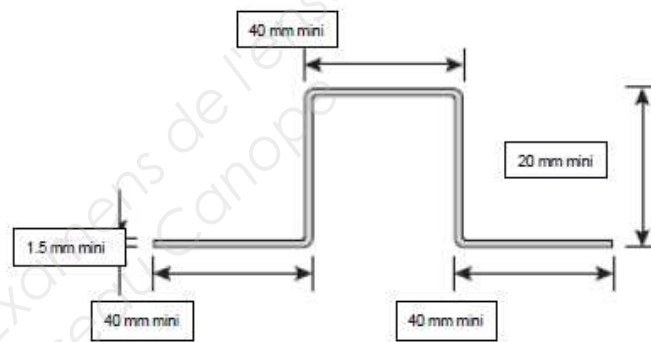
Figure 11 - Exemple d'ossature secondaire Oméga
