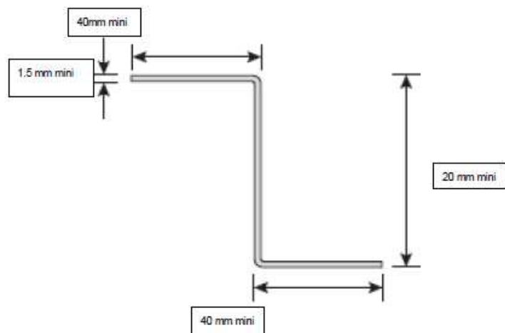
Figure 12 - Exemple d'ossature secondaire Z
