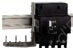
Bloc différentiel associé
