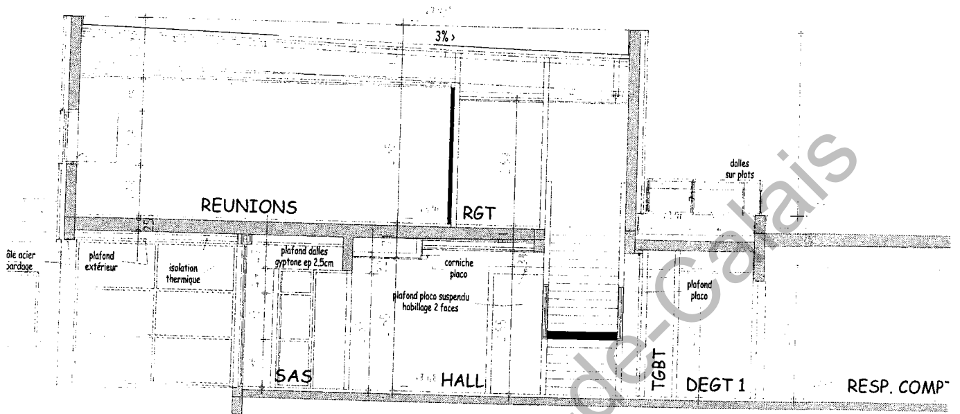
Coupe 4-4
